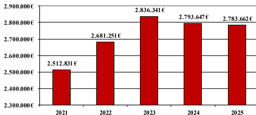
Umlagekraft
