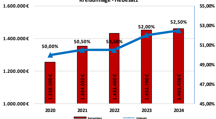
Kreisumlage - Hebesatz
